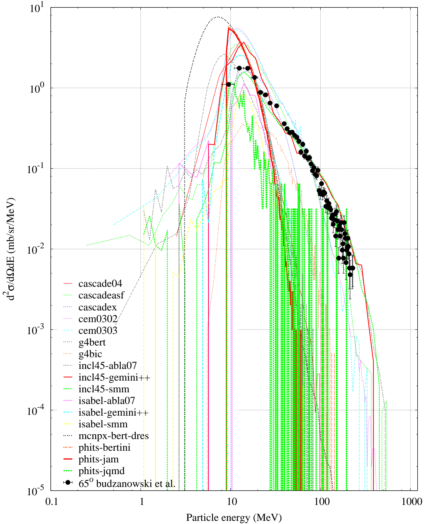
p (1200 MeV) + Au -- Triton spectrum
