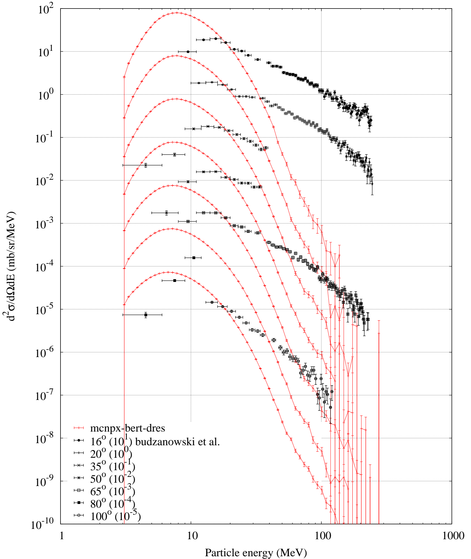
p (1200 MeV) + Au -- Triton spectrum
