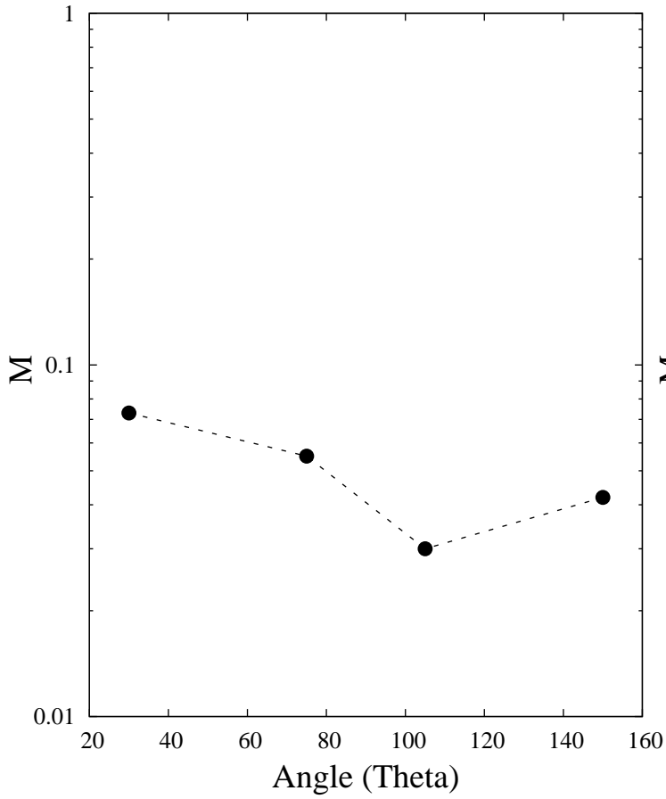
M factor - E_{\text{low}} (0-20 MeV)
