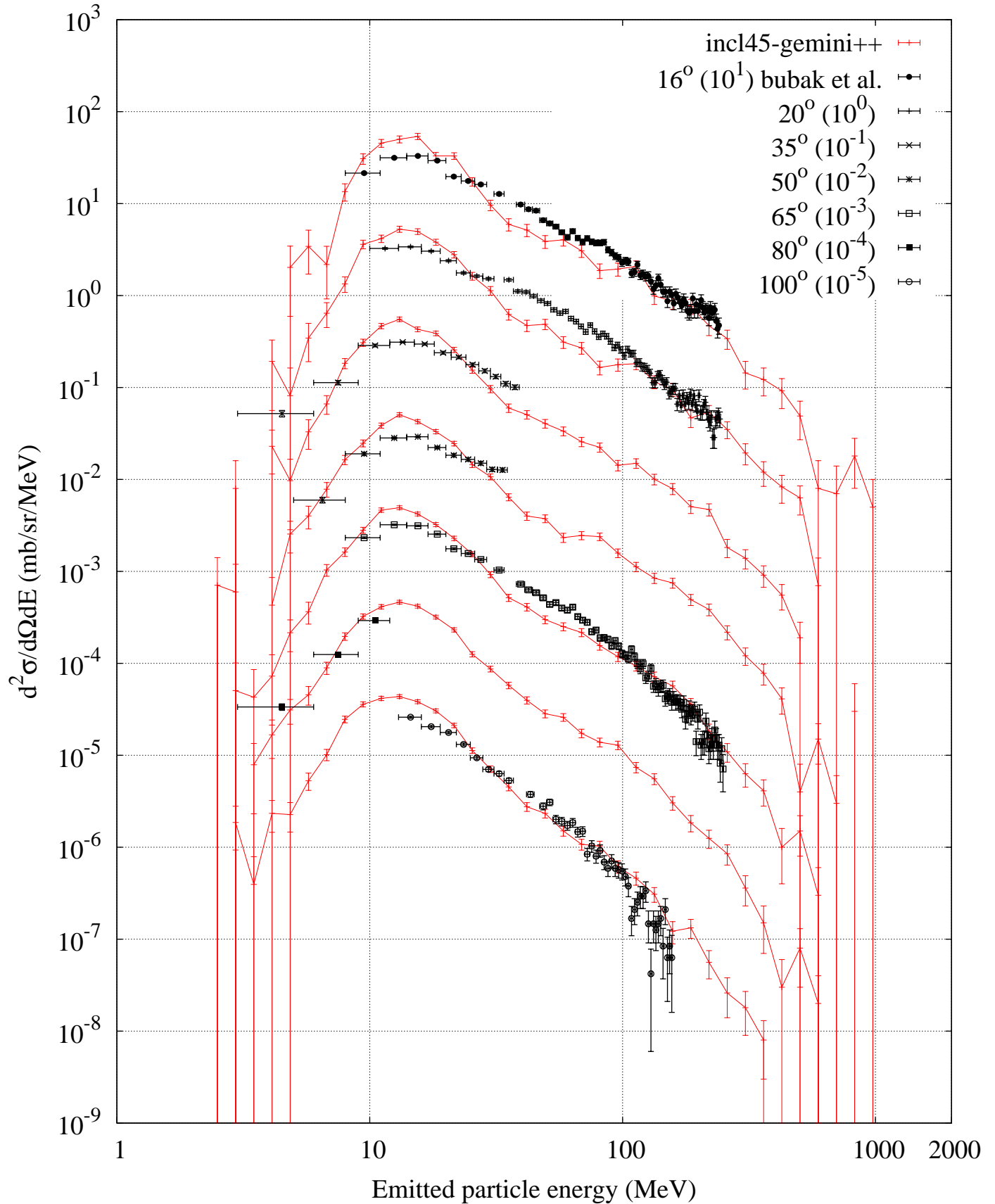
p (2500 MeV) + Au -- Tritium spectrum
