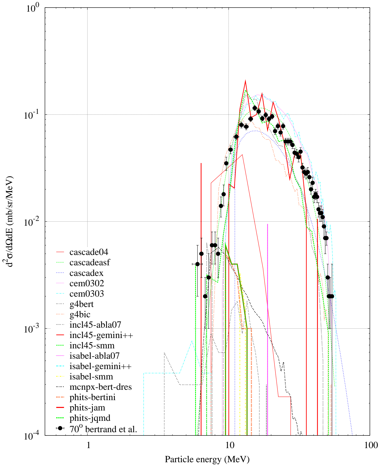
p (62 MeV) + Bi -- Triton spectrum
