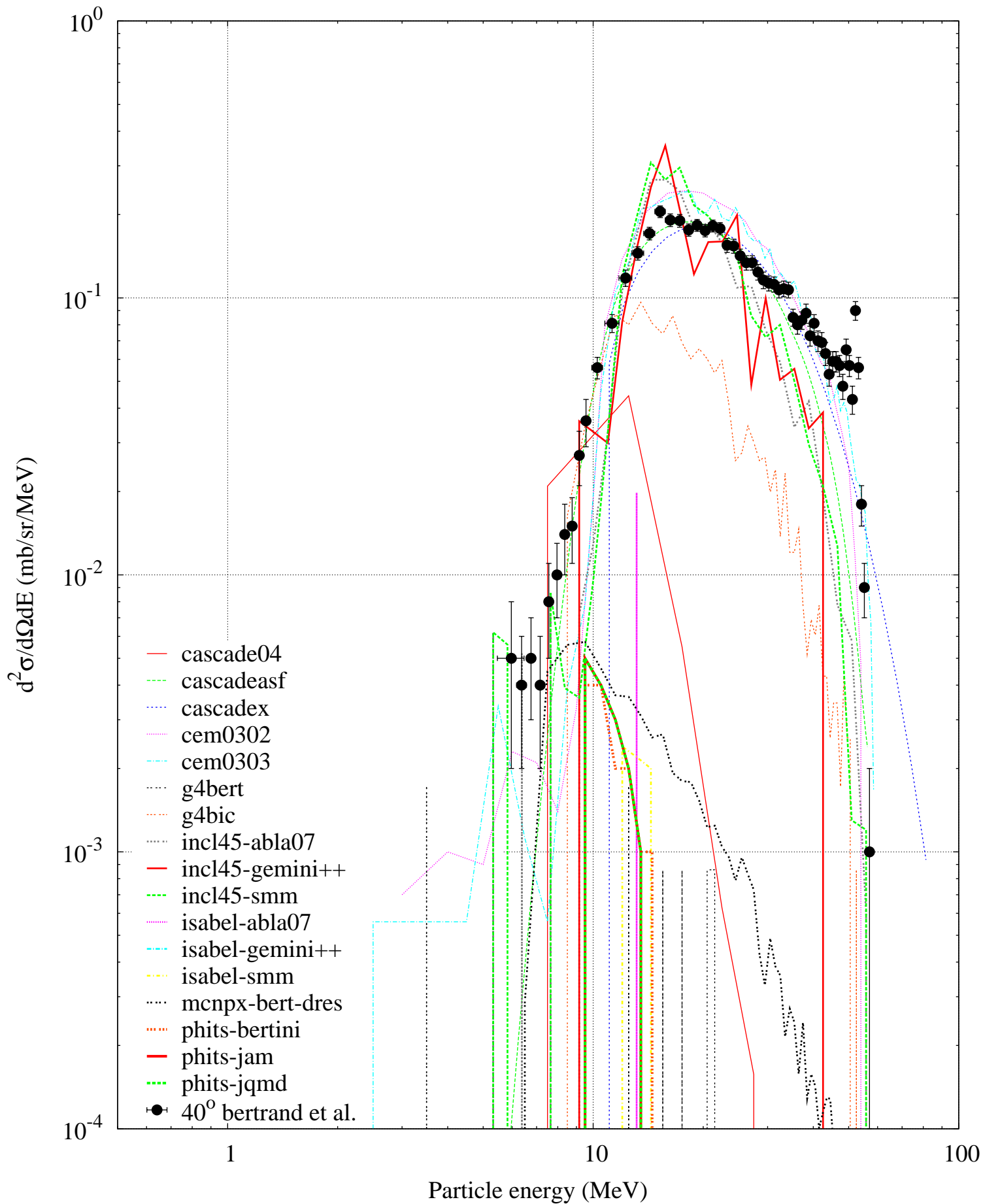
p (62 MeV) + Bi -- Triton spectrum
