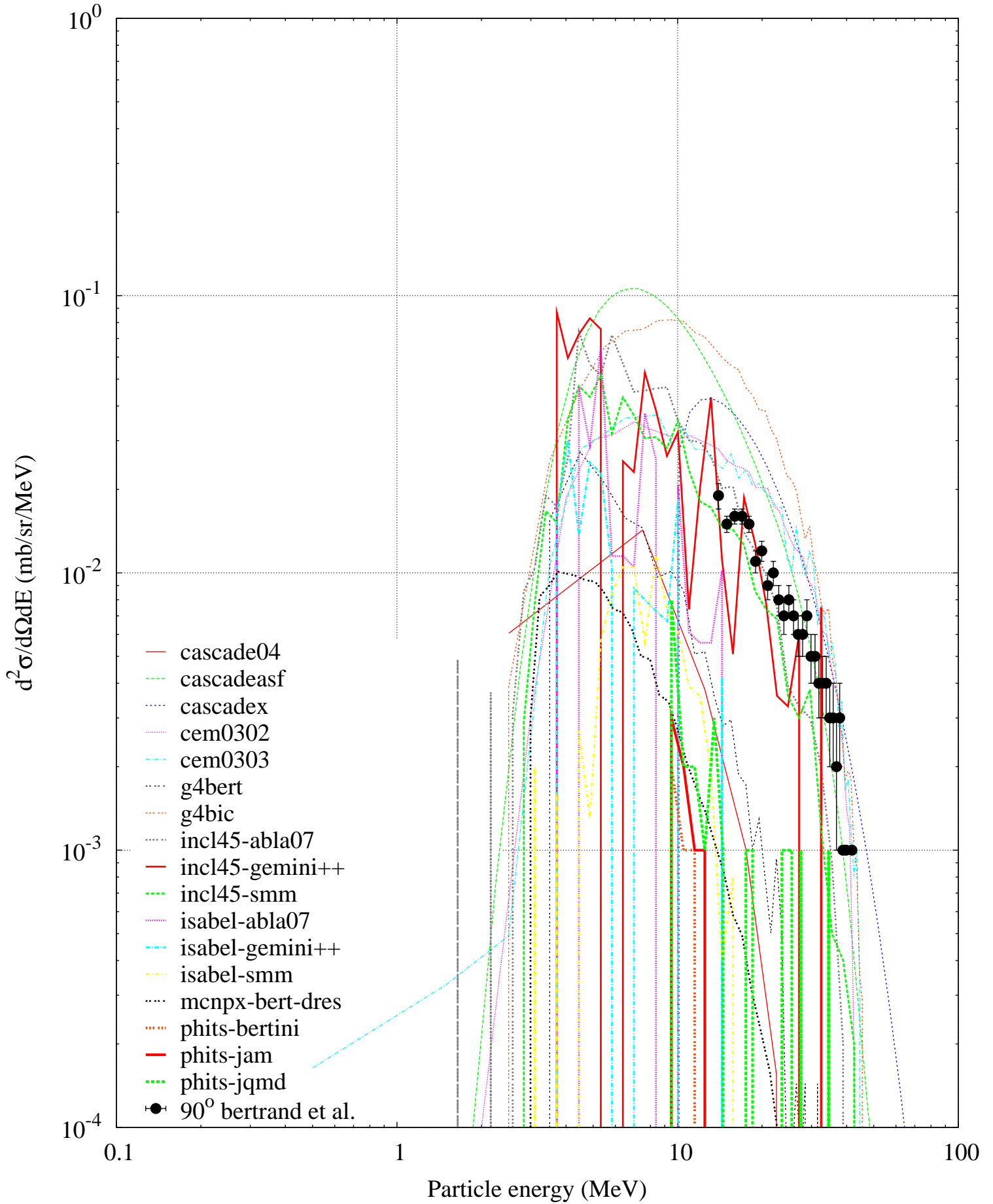
p (62 MeV) + Fe56 -- Triton spectrum
