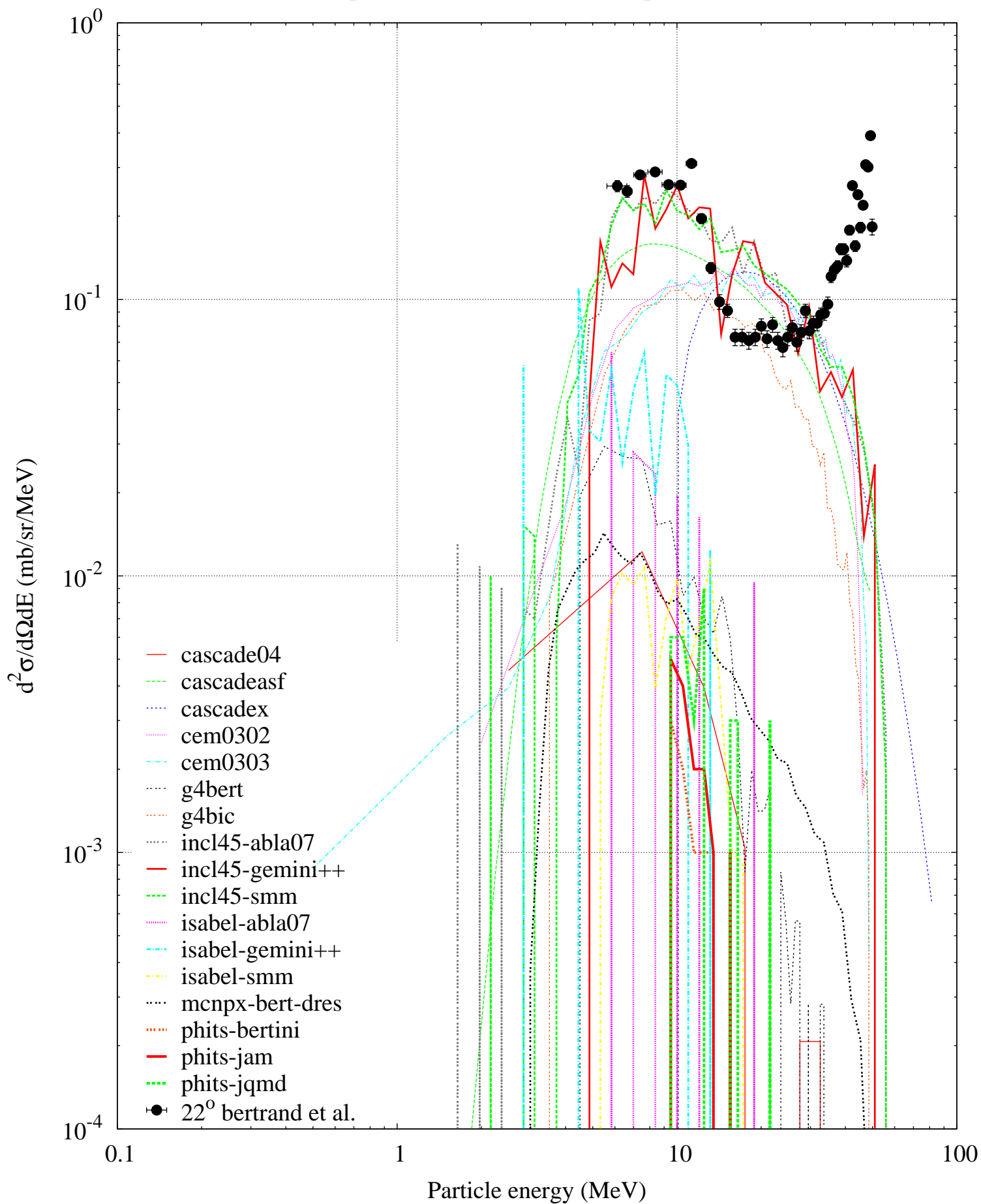
p (62 MeV) + Fe56 -- Triton spectrum
