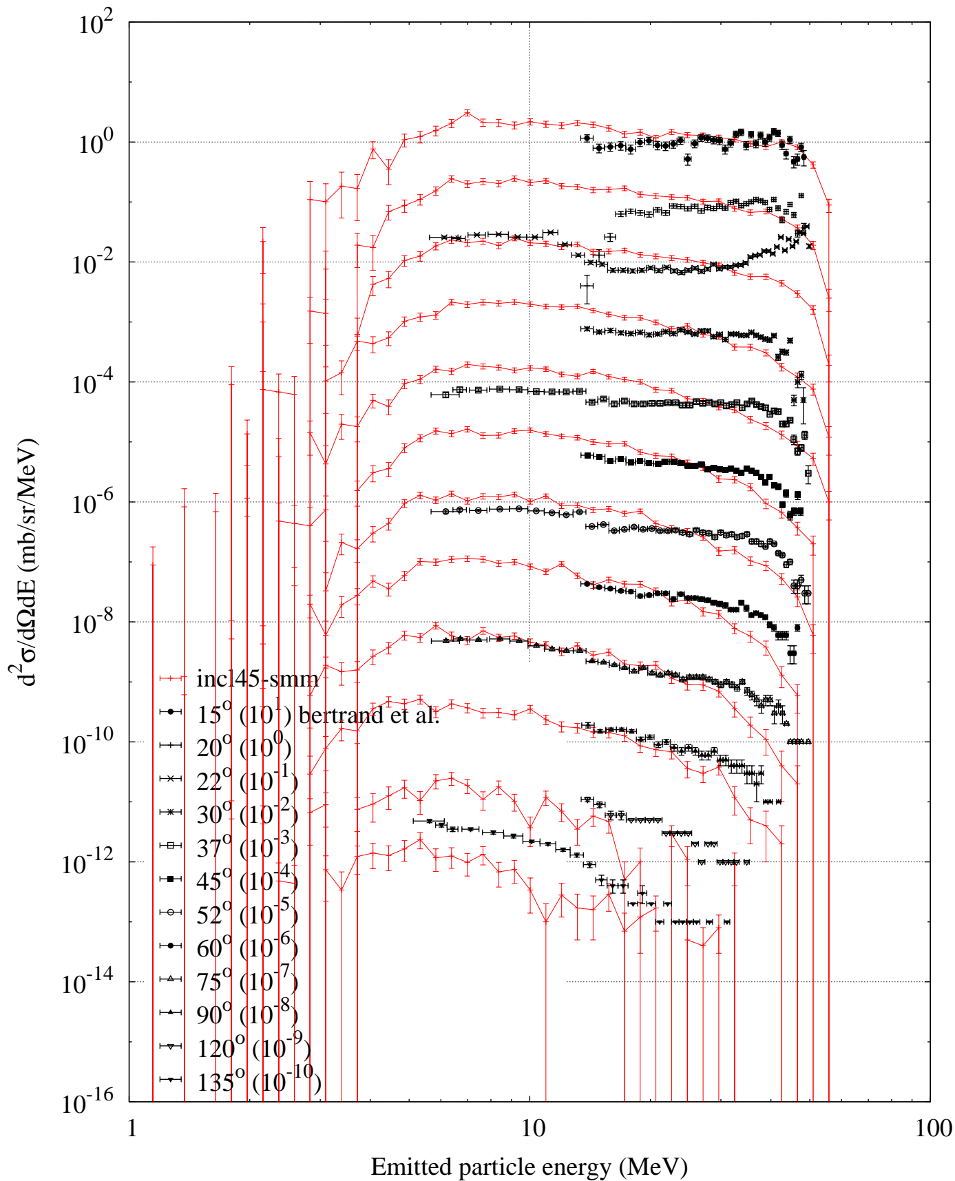
p (62 MeV) + Fe56 -- Tritium spectrum
