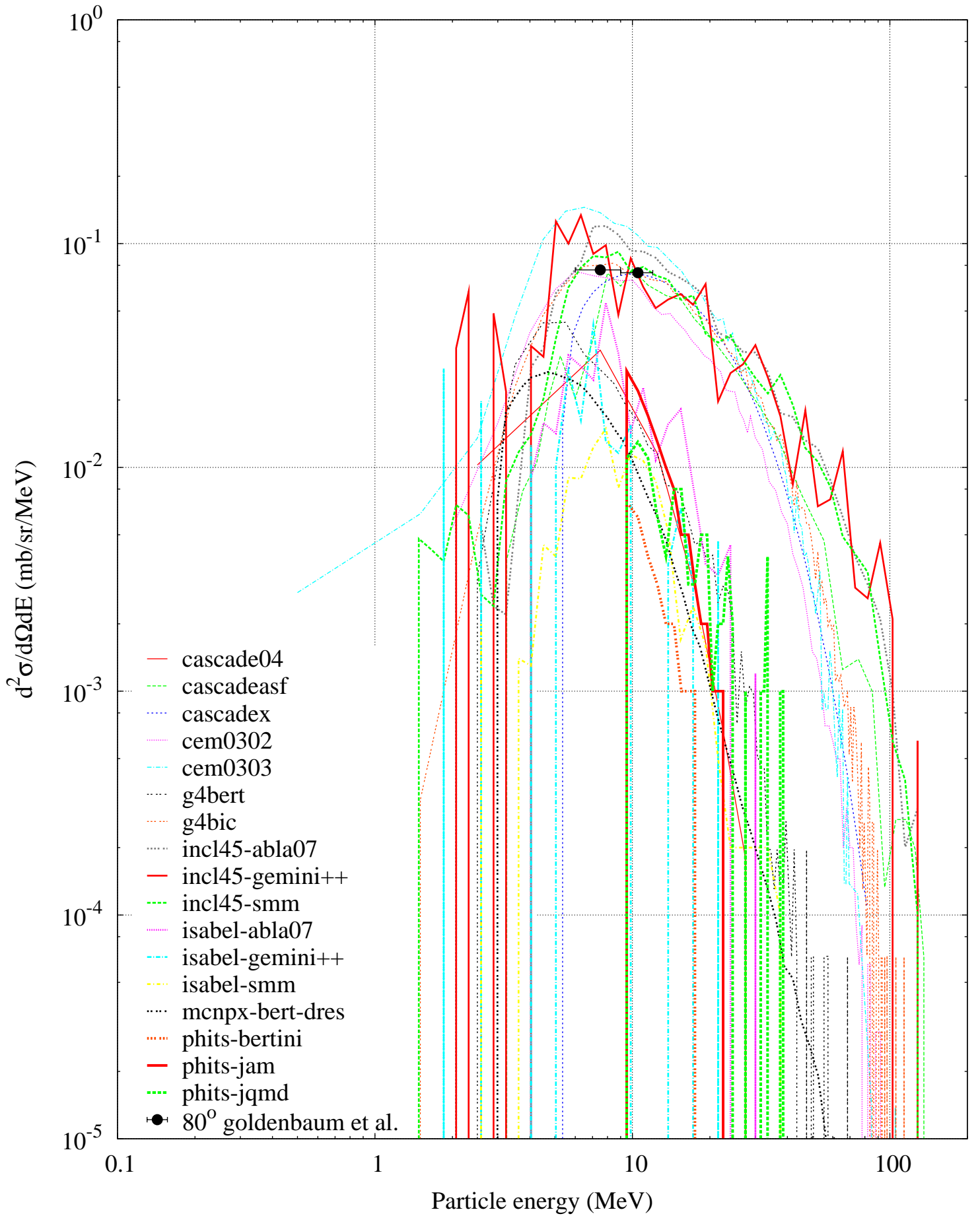
p (175 MeV) + Ni -- Triton spectrum
