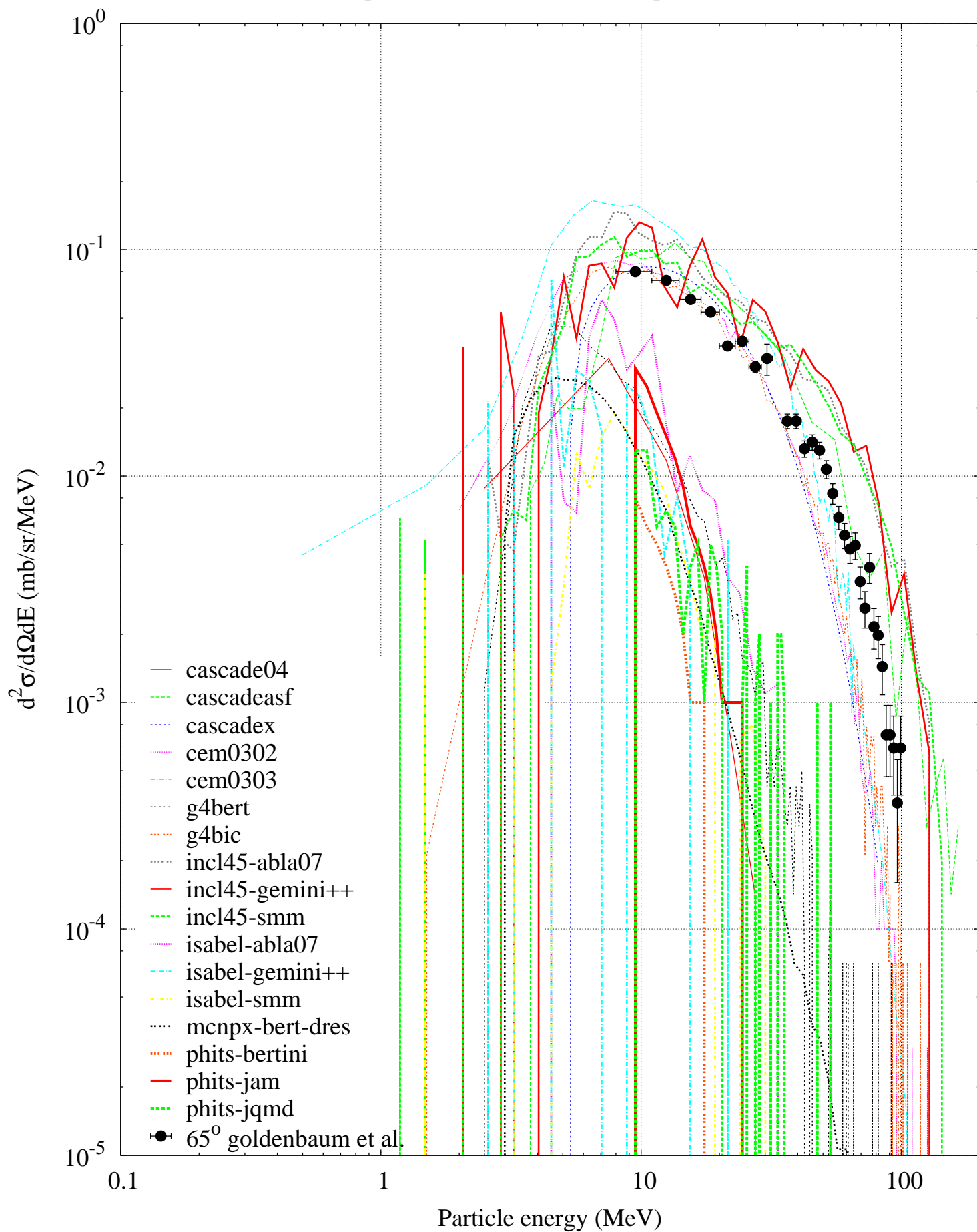
p (175 MeV) + Ni -- Triton spectrum
