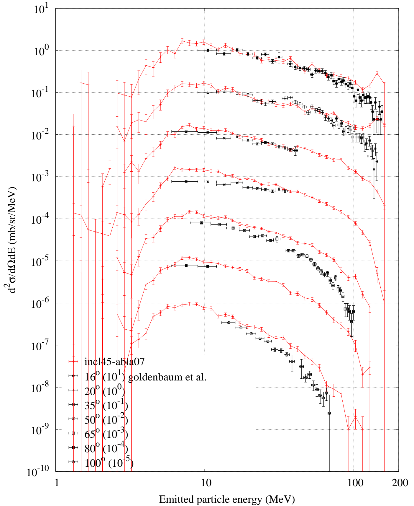
p (175 MeV) + Ni -- Tritium spectrum
