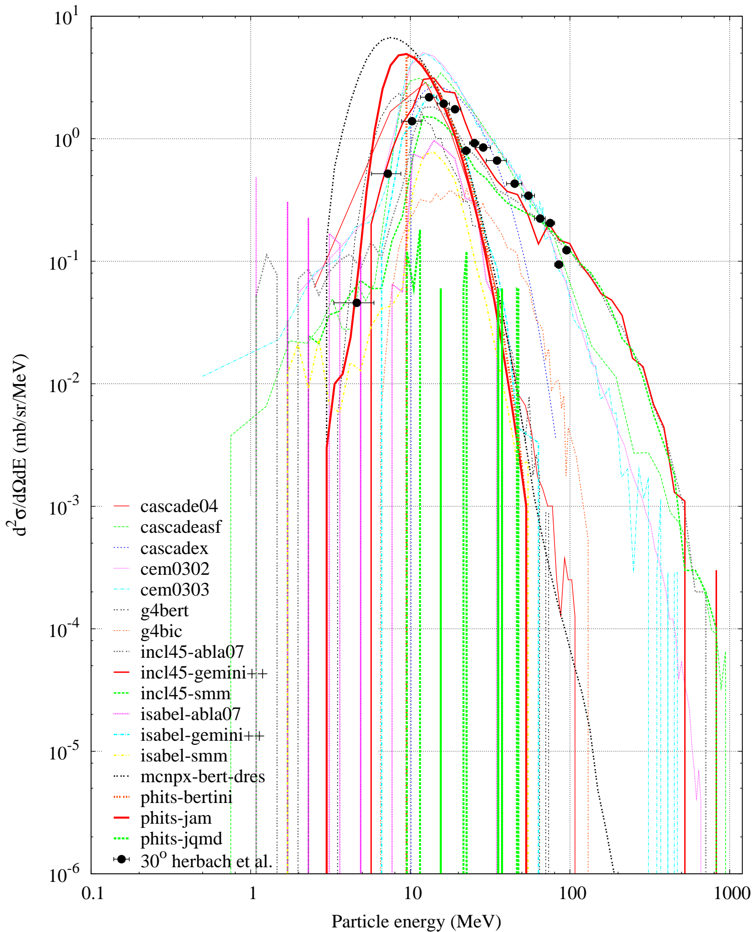
p (1200 MeV) + Ta -- Triton spectrum
