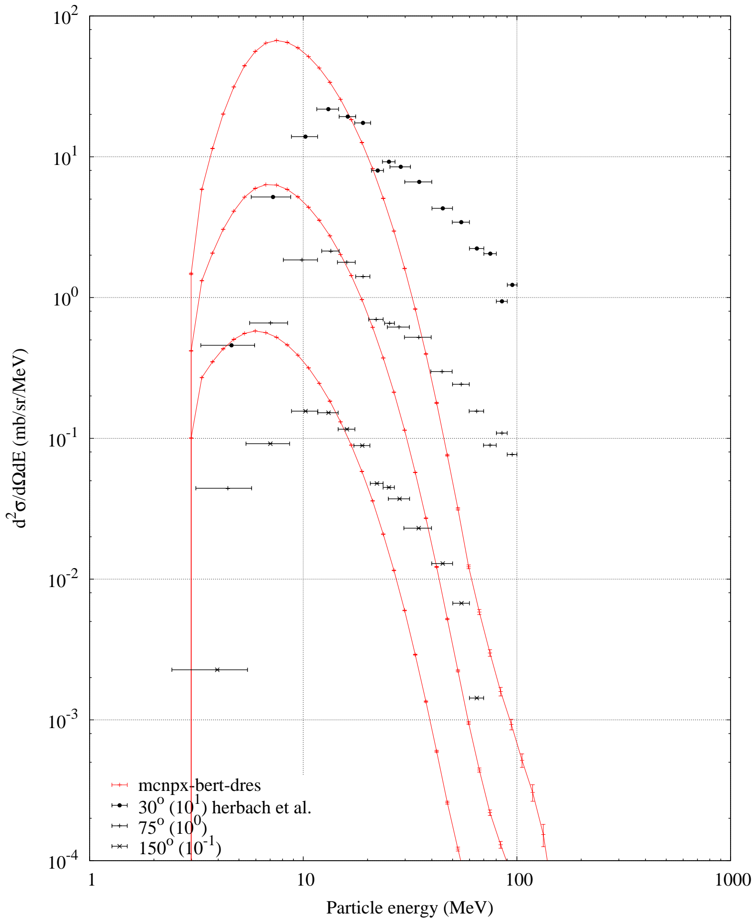
p (1200 MeV) + Ta -- Triton spectrum
