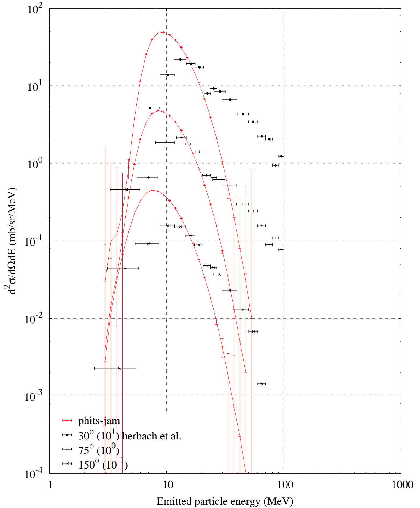
p (1200 MeV) + Ta -- Tritium spectrum
