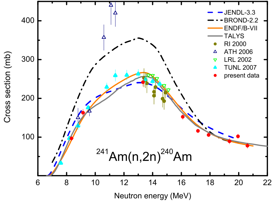
Figure 1: Mesures expérimentales de la section efficace de la réaction ^{241}\text{Am}(n,2n) obtenues à l'IRMM et comparées aux mesures et évaluations précédentes.
